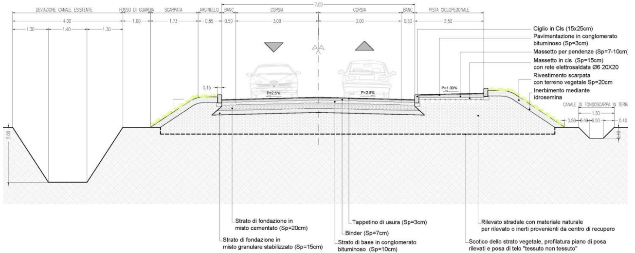
Figura 6: Sezione tipo in rilevato
