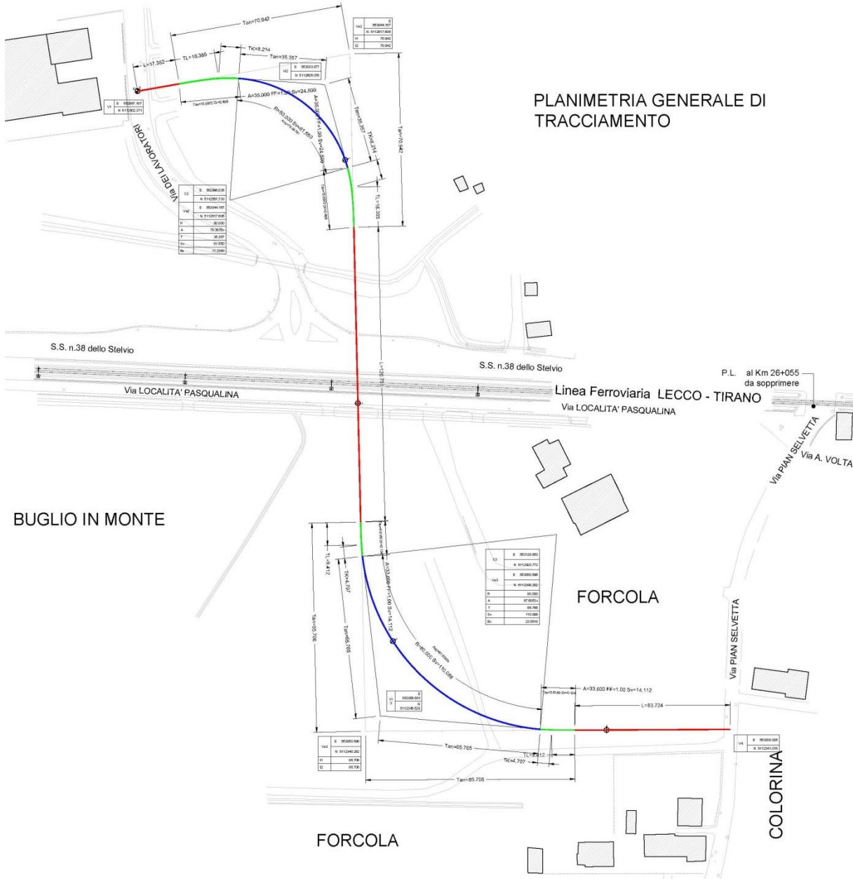
Figura 4: Tracciato planimetrico
