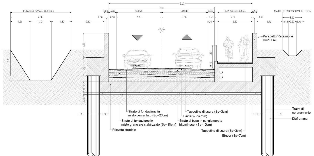
Figura 7: Sezione tipo in scavo
