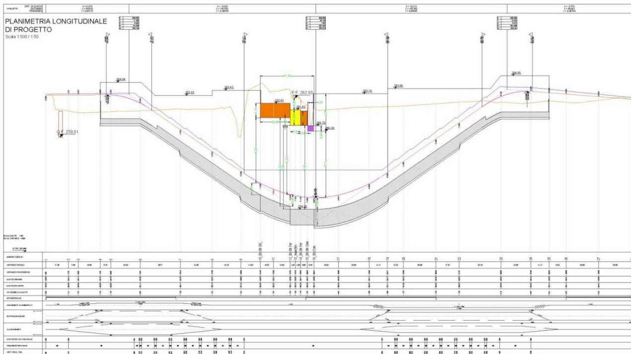
Figura 5: Tracciato altimetrico
