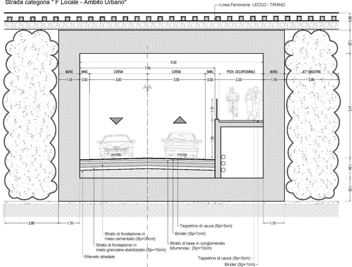
Figura 8: Sezione tipo nel sottovia
