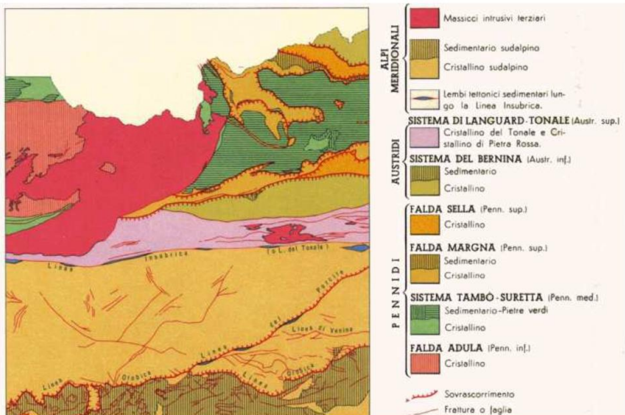
Figura 29: Schema strutturale della Valtellina
